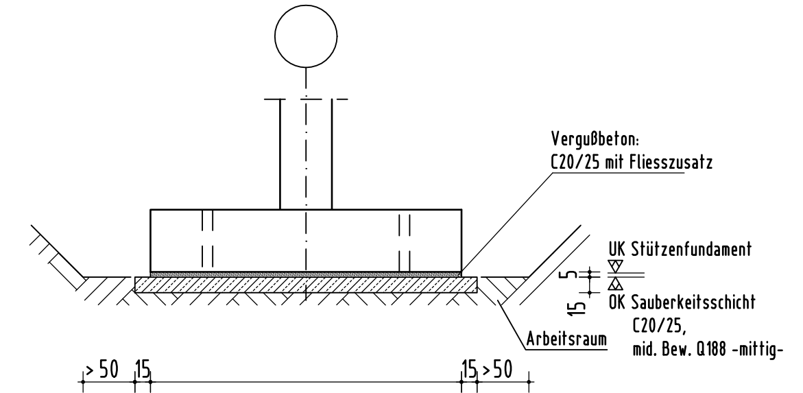
Stütze mit Fundamentplatte Regeldetail Arbeitsraum
